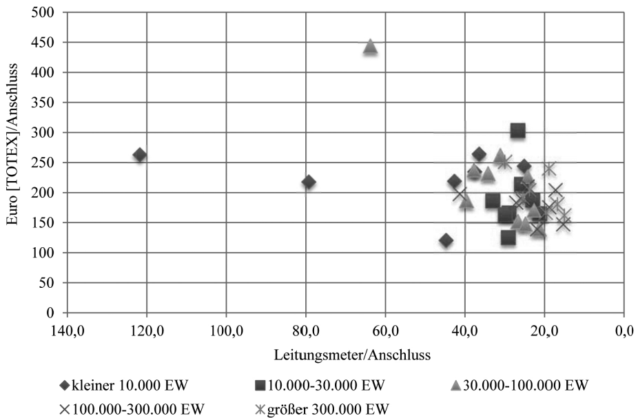
Abbildung 6: Kosten pro Anschluss und Meter Leitung pro Anschluss
